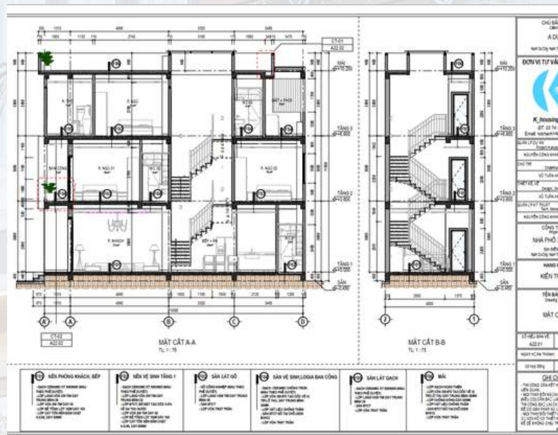
Thiết kế mặt cắt công trình
